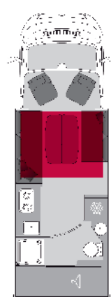
Lit de pavillon double non permanent
